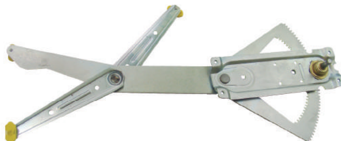
R-3342 E/D Máquina Reguladora Corsa 2P/ Pick-up Corsa ...2001 Nº Orig. 90.388.865 (LE) / 90.388.866 (LD)
