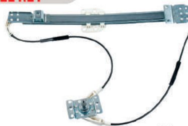
R-5140 E/D Máquina Reguladora Corcel II 2P 79...81 Nº Orig. BD8M-622.3201-A (LE) / BD8M-622.3200-A (LD)
