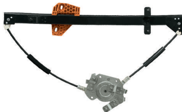
R-5218 E/D Máquina Reguladora
