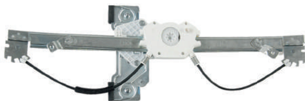
R-3362 E/D Máquina Reguladora Spin 4P TRS. 2012... C/ Motor - S/ Motor - Fixação Motor Mabuchi Nº Orig. 52.211.164 (LE) / 52.211.166 (LD)
