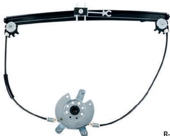
R-1435 E/D Máquina Reguladora Palio 2P / Pick-Up Strada 96... C/ Motor - S/ Motor - Fixação Motor Mabuchi Nº Orig. 46.736.840 (LE) / 46.736.841 (LD)
