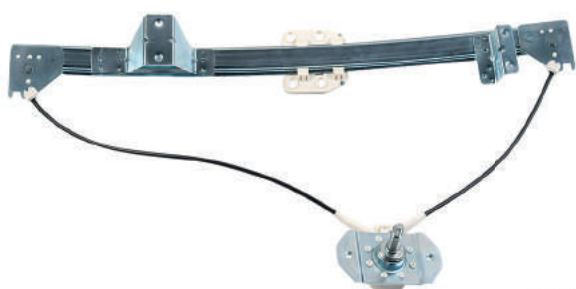
R-3346 E/D Máquina Reguladora Bonanza / Veraneio / A/C / D20A / D40 D12000 DNT. 91... Nº Orig. 52.255.121 (LE) / 52.255.122 (LD)
