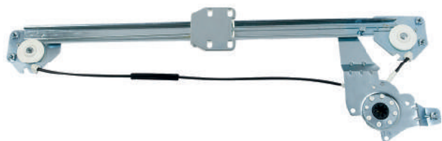
R-2613 E/D Máquina Reguladora Caminhão Volvo NL10/ NL12 90...94 Cabine Longa 24 Volts C/ Motor - S/ Motor - Fixação Motor Mabuchi Nº Orig. 8.123.551 (LE) / 8.123.550 (LD)
