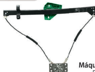
R-5142 E/D Máquina Reguladora Del Rey / Corcel II / Belina II 2P 82... Nº Orig. 80.NU.622.3201-A (LE) / 80.NU.622.3200-A (LD)
