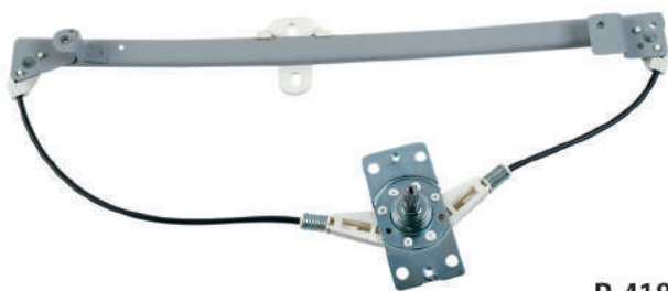
R-4185 E/D Máquina Reguladora Santana / Quantum / Versailles 4P TRS. 86...97 Nº Orig. ZBD.839.501.E (LE) / ZBC.839.502.D (LD)
