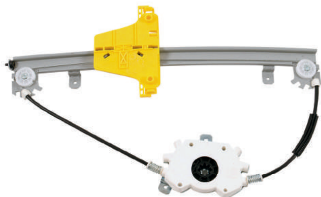
R-4133 E/D Máquina Reguladora Gol 4P / Voyage 4P GV / GVI DNT. 2008... C/ Motor - S/ Motor Fixação Motor Mabuchi Nº Orig. 5U4.837.399 (LE) / 5U4.837.400 (LD)
