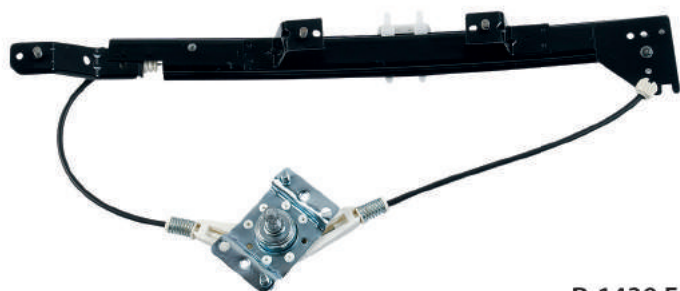
R-1439 E/D Máquina Reguladora Palio / Siena / Weekend 4P TRS. 96... 2012 Nº Orig. 46.446.911 (LE) / 46.446.910 (LD)
