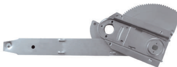
R-5222 E/D Máquina Reguladora F600 / F1000 / F4000 Caminhão 72...91 C/ Motor - S/ Motor - Fixação Motor Mabuchi Nº Orig. 89TU.81234W01B (LE) / 89TU.81234W00B (LD)
