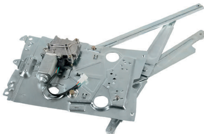
R-2613 E/D Máquina Reguladora Caminhão Volvo NL10/ NL12 90...94 Cabine Longa 24 Volts C/ Motor - S/ Motor - Fixação Motor Mabuchi Nº Orig. 8.123.551 (LE) / 8.123.550 (LD)
