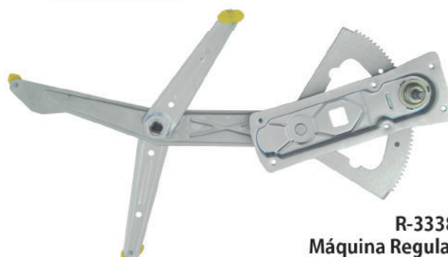
R-3336 E/D Máquina Reguladora Celta 2P ...2006 Pino Curto Nº Orig. 93.260.865 (LE) / 93.260.866 (LD)
