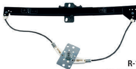
R-1419 E/D Máquina Reguladora Iveco Daily 35S14/ 40S16/ 55S14 2008... / Master 2008...2013 Nº Orig. 504.205.271 (LE) / 504.205.269 (LD)
