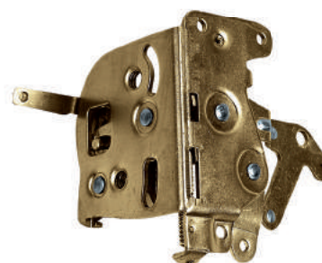
F-1440 E/D Fechadura Interna Uno / Prêmio / Elba 2P - Todos Nº Orig. 7.515.950 (LE) / 7.516.181 (LD)
