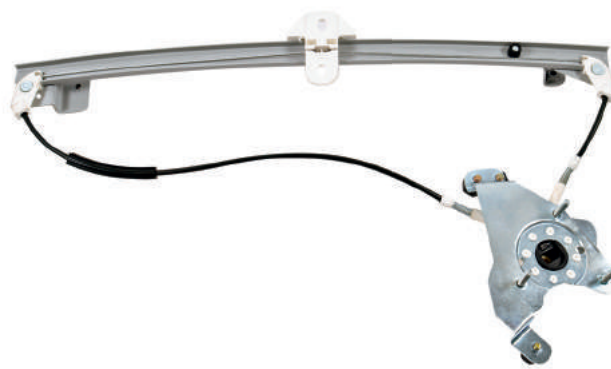
R-4194 E/D Máquina Reguladora Santana 4P TRS. 86...98 SM Somente sem Motor - Fixação Motor Carto Nº Orig. 327.839.501-5 (LE) / 327.839.502-5 (LD)
