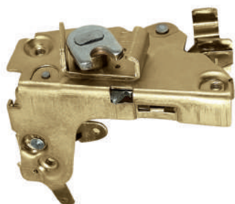
F-4498 E/D Fechadura Dianteira Kombi DNT. / Caminhão Volkswagen Todas Nº Orig. 231.837.015.1 (LE) / 231.837.016.1 (LD)
