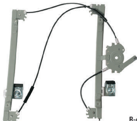
R-4191 E/D Máquina Reguladora Santana 4P DNT. 98... C/ Motor - S/ Motor - Fixação Motor Mabuchi Nº Orig. 327.837.501-3 (LE) / 327.837.502-3 (LD)
