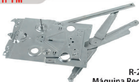
R-2612 E/D Máquina Reguladora Caminhão Volvo NL10/NL12 90... 94 Braço - Cabine Normal Nº Orig. 8.123.247 (LE) / 8.123.248 (LD)
