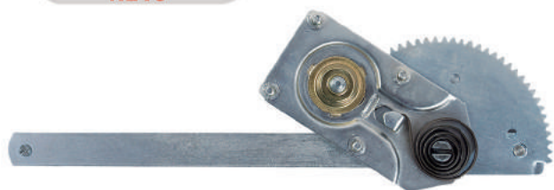
R-2612 E/D Máquina Reguladora Caminhão Volvo NL10/NL12 90... 94 Braço - Cabine Normal Nº Orig. 8.123.247 (LE) / 8.123.248 (LD)
