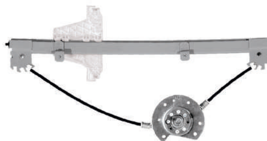
R-4401 E/D Máquina Reguladora Fox 4P TRS. Out-2009... Pino Longo Nº Orig. 5Z4.839.401D (LE) / 5Z4.839.402D (LD)
