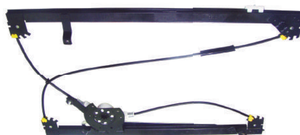
R-2614 E/D Máquina Reguladora Caminhão Volvo VM 2004... Todos C/ Motor - S/ Motor - Fixação Motor Mabuchi -12/24 Volts Nº Orig. 20.557.552 (LE) / 20.557.554 (LD)
