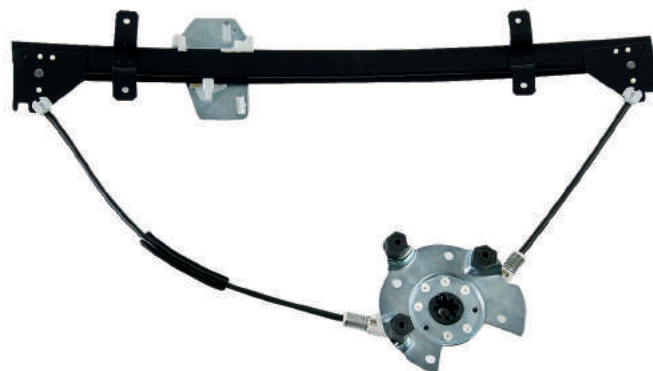
R-5230 E/D Máquina Reguladora Escort SW Zetec 4P 97... Pointer / Verona 93...96 DNT C/ Motor - S/ Motor - Fixação Motor Mabuchi Nº Orig. 97.AGA.23201AA (LE) / 97.AGA.23200AA (LD)
