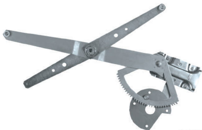
R-5233 E/D Máquina Reguladora Caminhão Cargo 81... 12V / 24 V / C/ Motor - S/ Motor - Fixação Motor Mabuchi Nº Orig. 81DBE23201AJ (LE) / 81DBE23200AJ (LD)
