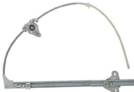
R-1450 E/D Máquina Reguladora Iveco Daily 35S14/ 40S16/ 55S14 2008... Master 2008... Somente sem Motor - Fixação Motor Original Nº Orig. 504.173.868 (LE) / 504.173.869 (LD)
