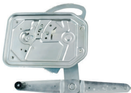
R-2607 E/D Máquina Reguladora Caminhão Scania Série 4 114 / 124 / T/R 98... C/ Motor - S/ Motor - Fixação Motor Original Nº Orig. 1.442.294 SM (LE) / 1.442.295 SM (LD)
