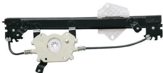
R-7505 E/D Máquina Reguladora Sandero 4P TRS. 2008... C/ Motor - S/ Motor - Fixação Motor Mabuchi Nº Orig. 82.006.037.95 (LE) / 82.006.038.10 (LD)
