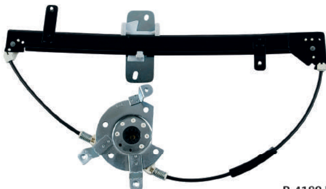
R-4189 E/D Máquina Reguladora Gol / Parati GII/ GIII/ GIV 4P TRS. 98...2007 C/ Motor - S/ Motor - Fixação Motor Mabuchi Nº Orig. 373.839.501.B.SM (LE) / 373.839.502.B.SM (LD)
