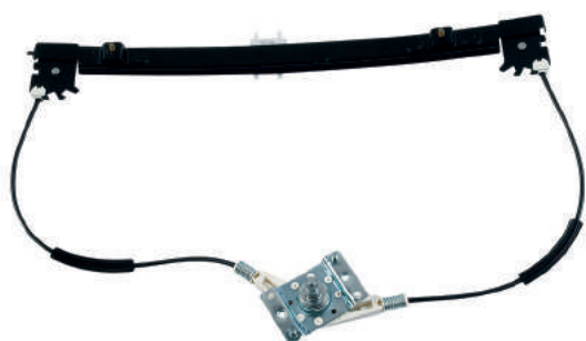
R-1437 E/D Máquina Reguladora Palio 2P / Pick-up Strada 96... Nº Orig. 46.446.909 (LE) / 46.446.908 (LD)
