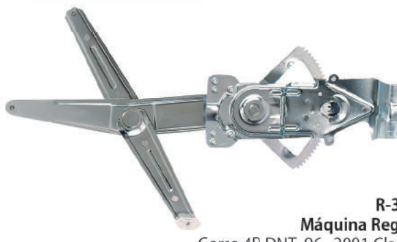
R-3335 E/D Máquina Reguladora Agile 4P TRS. 2009... C/ Motor - S/ Motor - Fixação Motor Mabuchi Nº Orig. 94.700.279 (LE) / 94.700.280 (LD)
