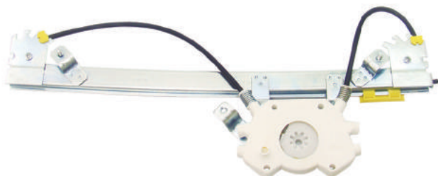
R-1429 E/D Máquina Reguladora Uno 4P TRS. 2010... C/ Motor - S/ Motor - Fixação Motor Mabuchi Nº Orig. 518.358.880 (LE) / 518.358.879 (LD)
