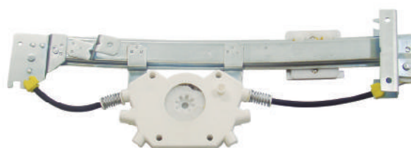
R-3349 E/D Máquina Reguladora Corsa Classic 4P TRS. 96... C/ Motor - S/ Motor - Fixação Motor Mabuchi Nº Orig. 93.253.441 (LE) / 93.253.442 (LD)
