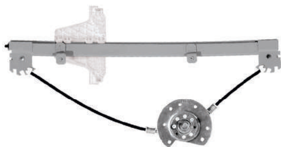
R-4398 E/D Máquina Reguladora Fox 4P TRS. 2003... Set-2009 Pino Curto Nº Orig. 5Z4.839.401 (LE) / 5Z4.839.402 (LD)
