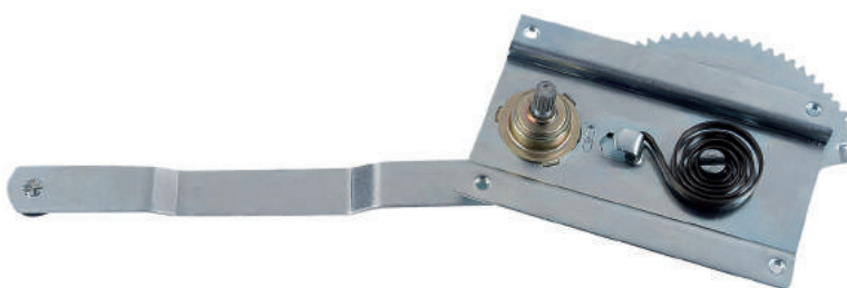
R-2621 E/D Máquina Reguladora Toyota 82...83 - Pino Estriado Nº Orig. 6980.298.002A (LE) / 6980.198.002A (LD)
