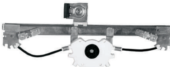
R-3335 E/D Máquina Reguladora Agile 4P TRS. 2009... C/ Motor - S/ Motor - Fixação Motor Mabuchi Nº Orig. 94.700.279 (LE) / 94.700.280 (LD)
