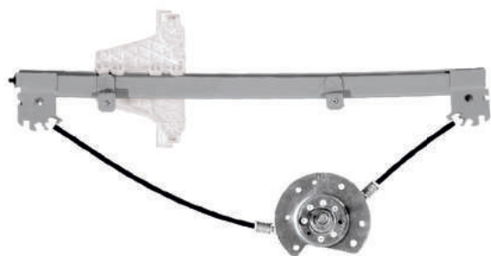
R-4400 E/D Máquina Reguladora Fox 4P DNT. Out-2009... Pino Longo Nº Orig. 5Z4.837.401G (LE) / 5Z4.837.402G (LD)
