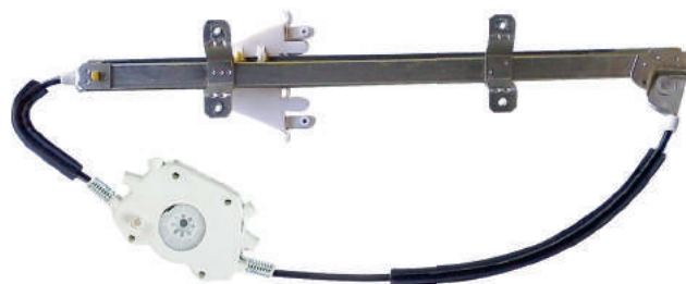
R-5236 E/D Máquina Reguladora Ford Cargo 2011... 12/24 V/ C/ Motor - S/ Motor - Fixação Motor Mabuchi Nº Orig. 3C46.E23201.BE (LE) / 3C46.E23200.BE (LD)
