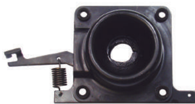
F-2917 E/D Fecho do Capô Inferior Caminhão Volvo NH 99...2006 Nº Orig. 20.565.618 (LE) / 20.565.619 (LD)
