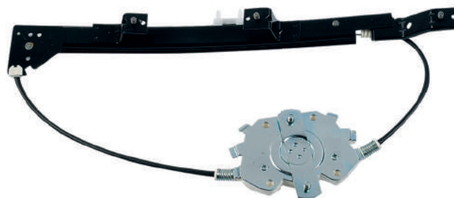
R-1434 E/D Máquina Reguladora Palio / Siena 96...2011 Weekend 4P TRS. 96... C/ Motor - S/ Motor - Fixação Motor Mabuchi Nº Orig. 46.446.911 (LE) / 46.446.910 (LD)
