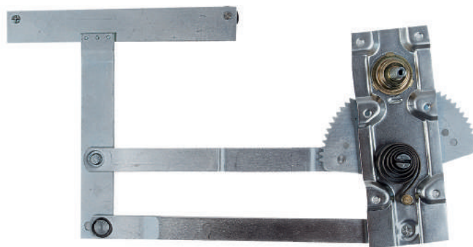
R-2602 E/D Máquina Reguladora Caminhão Scania L110 / 111 75...80 Nº Orig. 236.255 (LE) / 236.256 (LD)
