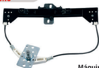
R-1420 E/D Máquina Reguladora Uno / Prêmio / Elba 2P Nº Orig. 50.006.099 (LE) / 50.006.098 (LD)
