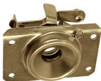
F-4203-I Fecho de Capô Sedan 1300-1500 71...81 Inferior Nº Orig. 113.853.509.1 (Inf.)
