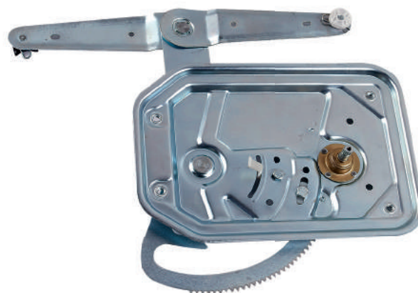
R-2606 E/D Máquina Reguladora Caminhão Scania Série 4 98... Nº Orig. 1.366.847 (LE) / 1.366.848 (LD)
