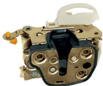
F-3355 E/D Fechadura Corsa 2/4P DNT ...2001 Classic 96... Nº Orig. 90.452.381 (LE) / 90.452.382 (LD)
