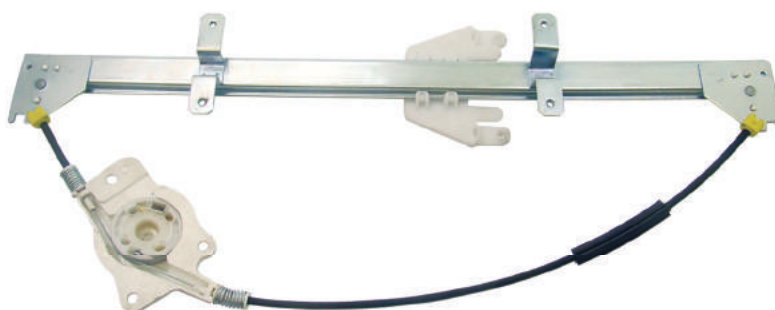
R-5237 E/D Máquina Reguladora Ford Cargo 2011... Somente sem Motor – Fixação Motor Original Nº Orig. 3C4.6E2.320.1BE (LE) / 3C4.6E2.320.0BE (LD)
