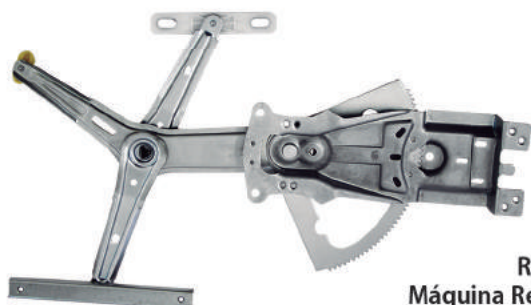
R-3364 E/D Máquina Reguladora Vectra 4P DNT. 96...2004 Somente sem Motor - Fixação Motor Original Nº Orig. 93.329.516 (LE) / 93.329.517 (LD)
