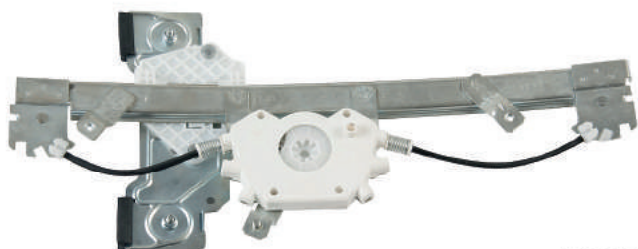
R-3360 E/D Máquina Reguladora Onix 4P TRS. 2012... Prisma 2013... C/ Motor - S/ Motor - Fixação Motor Mabuchi Orig. 52.039.026 (LE) / 52.039.027 (LD)
