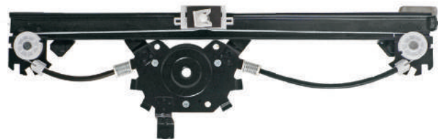
R-1426 E/D Máquina Reguladora Idea TRS. - Todos C/ Motor - S/ Motor - Fixação Motor Mabuchi Nº Orig. 51.783.849 (LE) / 51.783.847 (LD)
