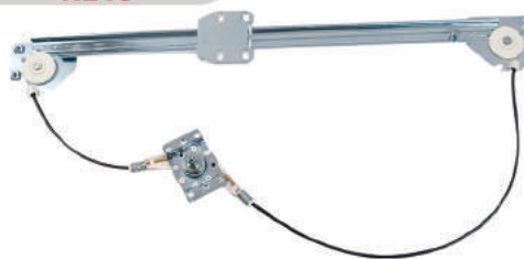
R-2611 E/D Máquina Reguladora Caminhão Volvo NL10/NL12 90... 94 Cabine Longa Nº Orig. 8.123.657 (LE) / 8.123.658 (LD)
