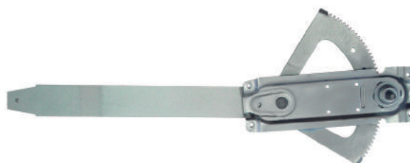
R-3322 E/D Máquina Reguladora Monza 2P - Cremalheira ...83 Nº Orig. 90.035.485 (LE) / 90.035.486 (LD)
