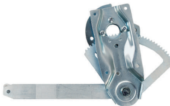
R-5232 E/D Máquina Reguladora Escort SW - Zetec 4P 97... Pointer / Verona 93...96 TRS. C/ Motor - S/ Motor - Fixação Motor Mabuchi Nº Orig. 97.AGA.27001BA (LE) / 97.AGA.27000BA (LD)
