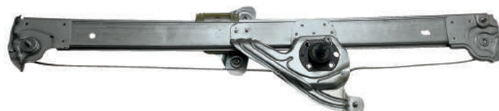
R-2308 E/D Máquina Reguladora Caminhão Mercedes Benz Accelo 815 / 1016 2012... Nº Orig. 979.720.11.46 (LE) / 979.720.12.46 (LD)
