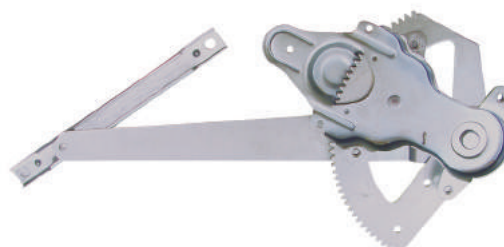
R-3363 E/D Máquina Reguladora S10 4P TRS. 2012... Especial (O vidro desce até o final do curso) C/ Motor - S/ Motor - Fixação Motor Mabuchi Nº Orig. 05.483.148 (LE) / 05.483.149 (LD)
